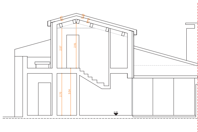
Sezione AA
