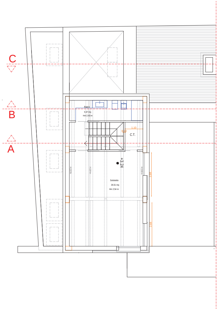
Piano primo
