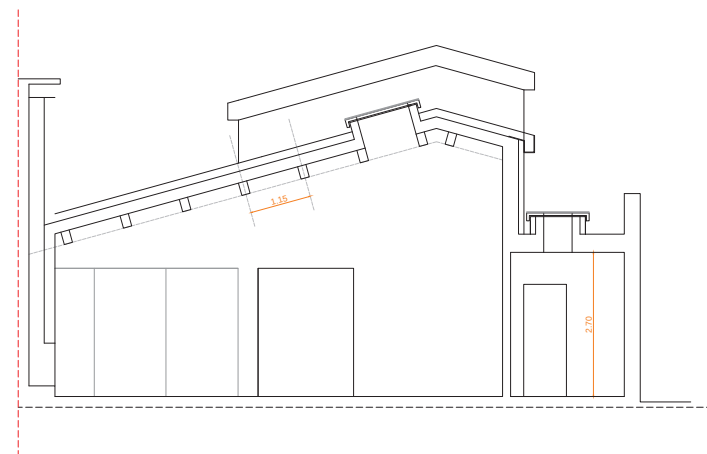
Sezione CC
