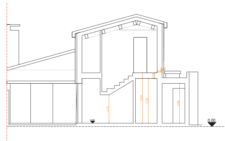
Sezione AA
