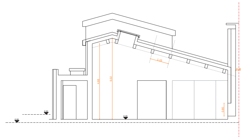
Sezione CC
