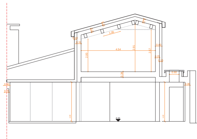
Sezione BB
